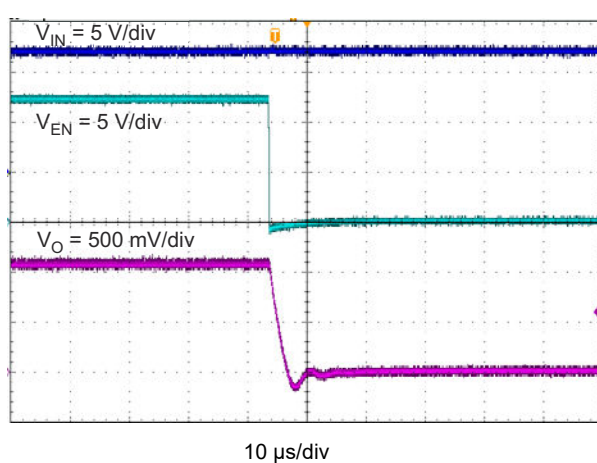
图 8-17. TPS562201 Shutdown Relative to EN
