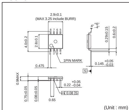
MSOP8
