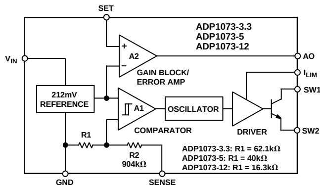
ADP1073-3.3, 5, 12
