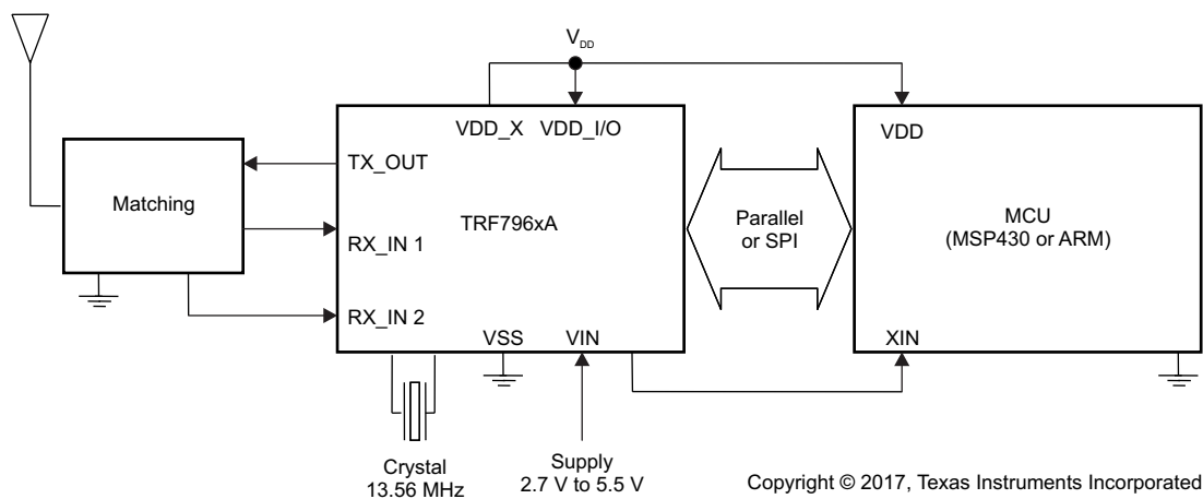
图 1-1. 应用框图
