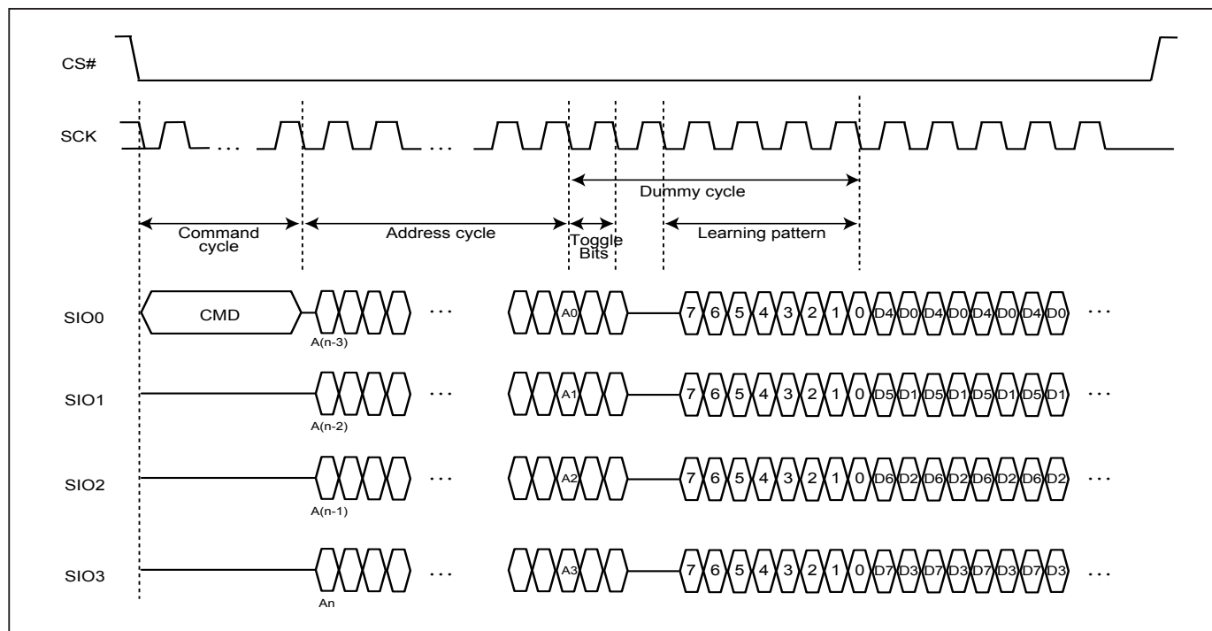
Figure 51. DTR4IO (DC=6)
