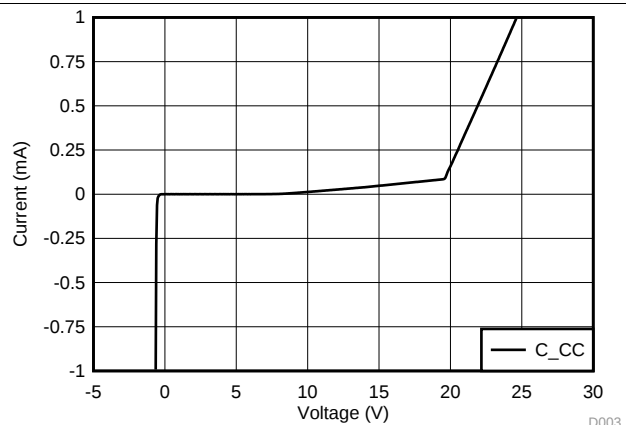
图 24. C_CC IV Curve
