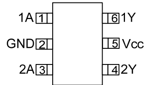
SOT363
