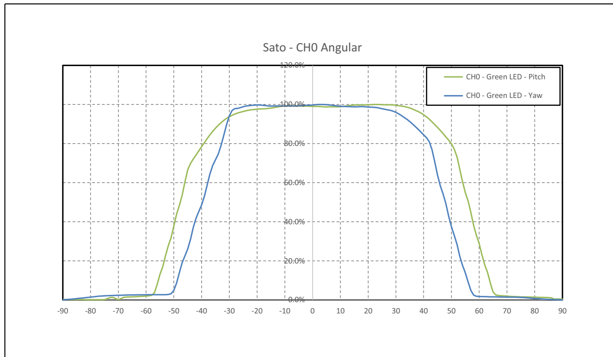
Figure 13: Typical ALS Angular Response
