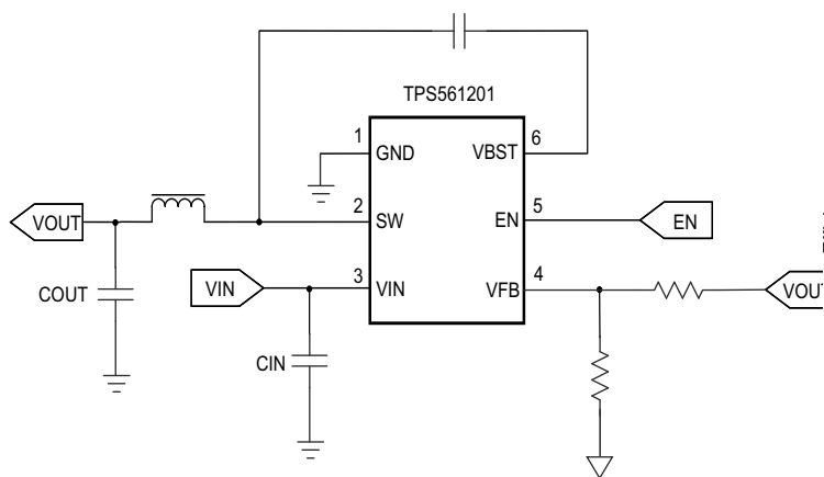
简化原理图
