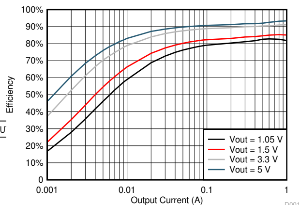
TPS561201 效率
