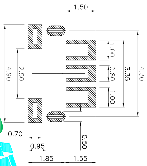
PCB Layout(Pattern side)
