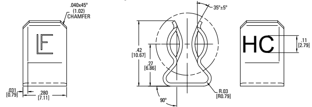
SMT Clip-124060
