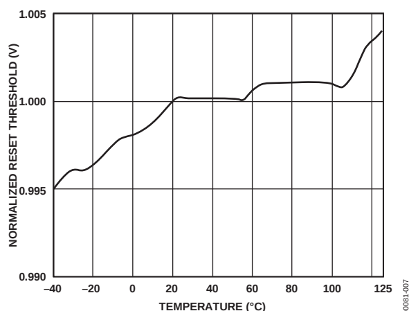
图8.归一化复位阈值与温度的关系 ( V_{CC} 下降)
