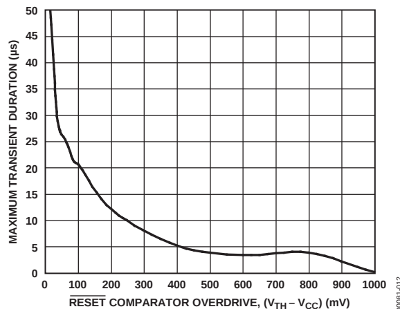
图7.最大瞬变持续时间与RESET比较器过驱的关系
