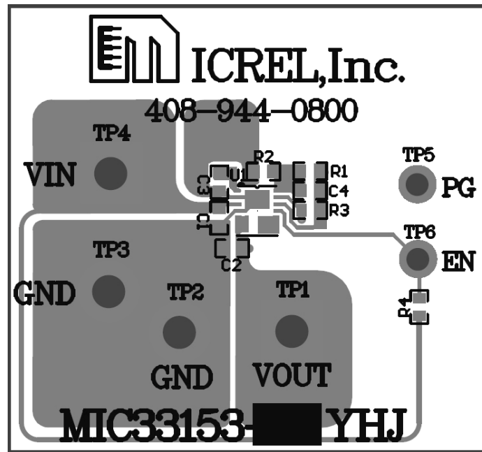
Top Layer
