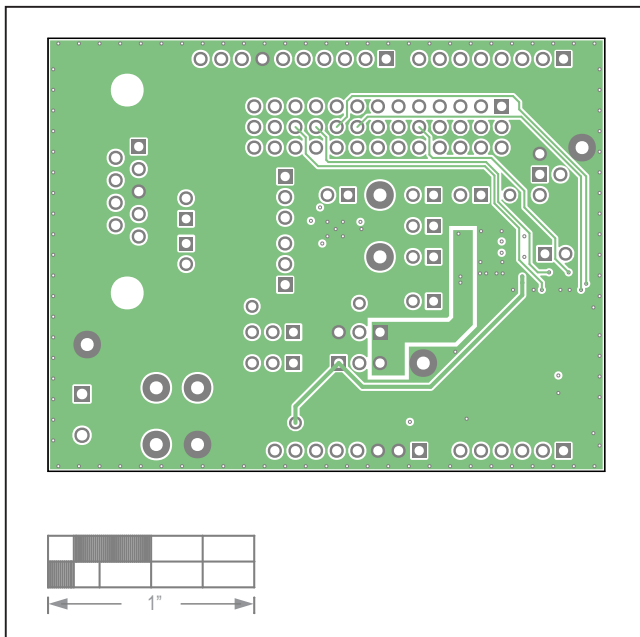
MAX33015E Shield—Internal 3
