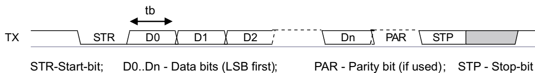
图 8-11. UART 数据帧
