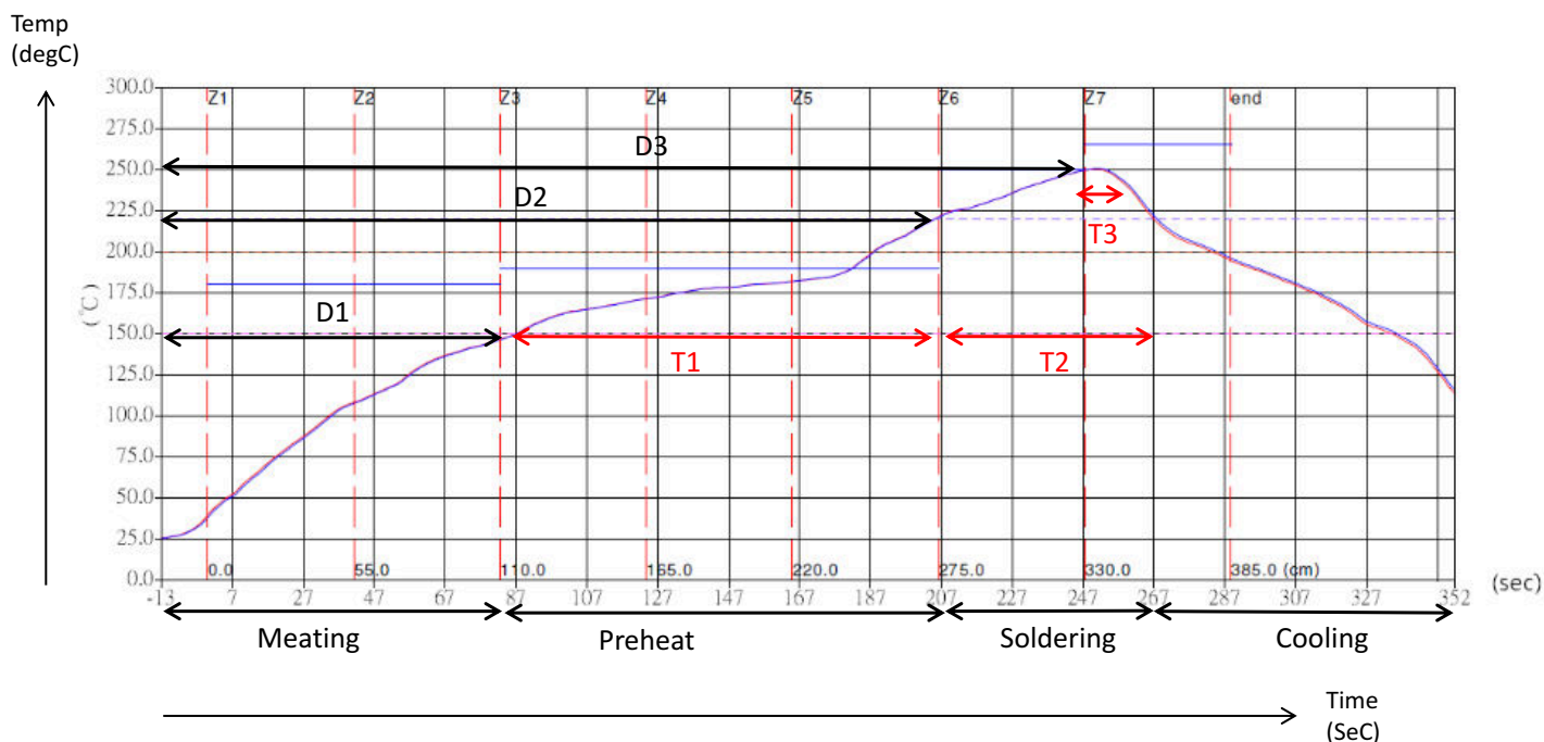
图 10-7. WiLink 8 模块的回流焊曲线
