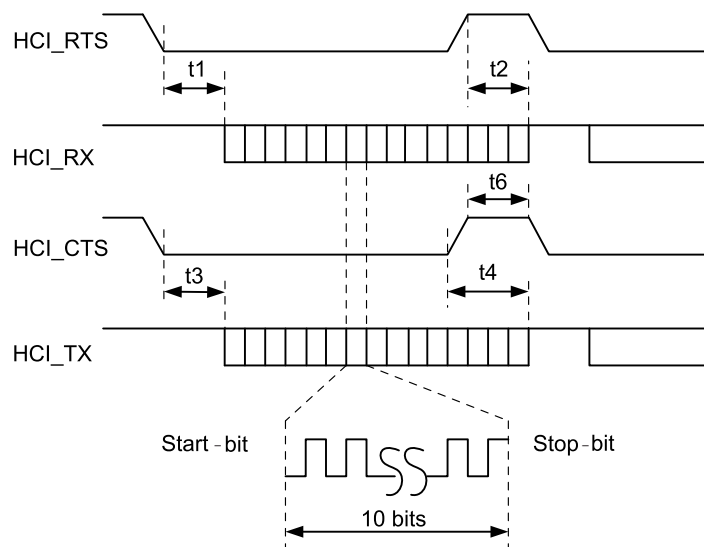
图 8-10. UART 时序图
