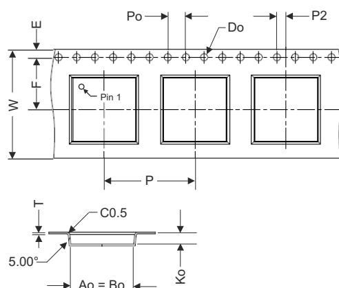
图 12-2. 卷带规格
