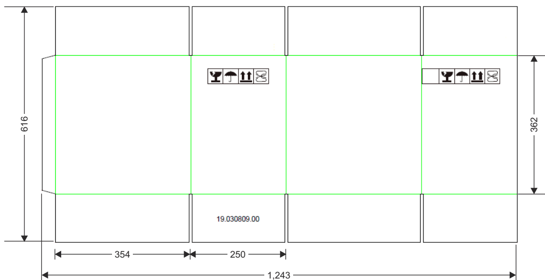
图 12-5. 装运箱
