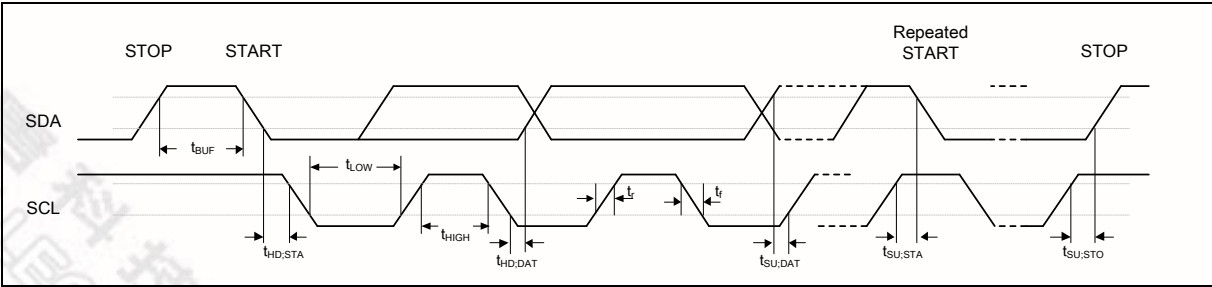
图 8-4 I2C 时序图
