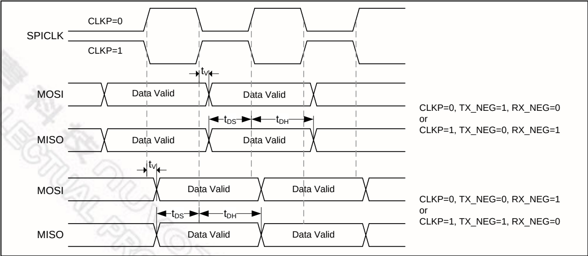
图 8-5 SPI 主机模式时序图
