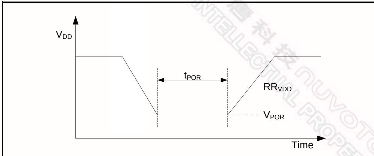
图 8-3 上电条件
