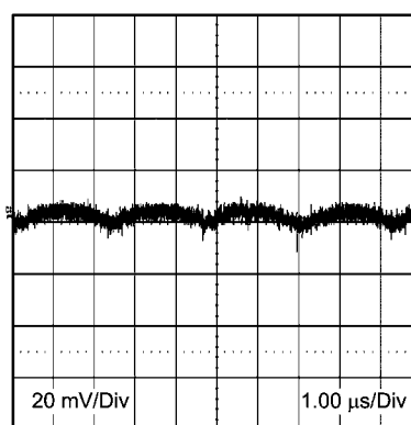
输出纹波
