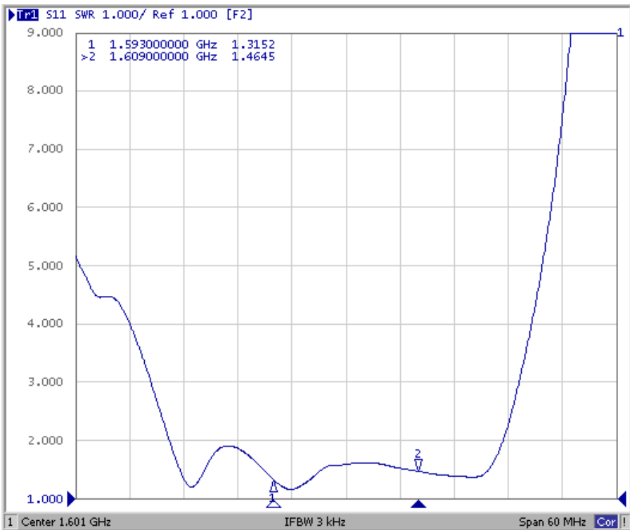
S11 VSWR
