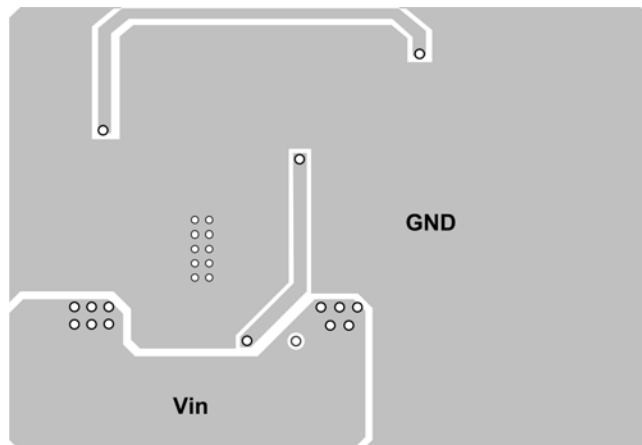
Bottom Layer
