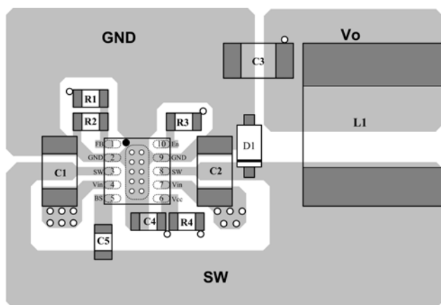
Top Layer
