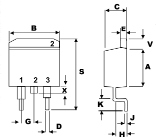
TO-263 (D2-PAK)
