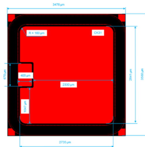
DIE OUTLINE
