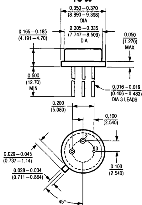
LT581 TO-39
