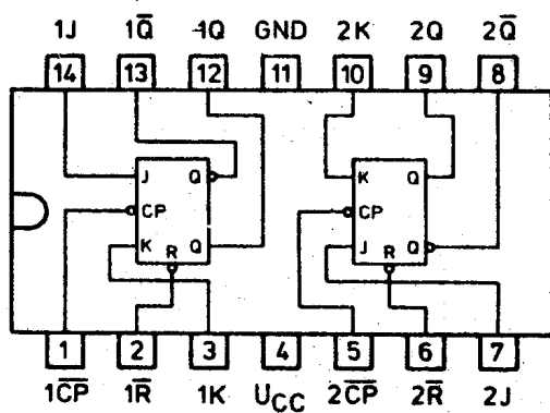
7473
