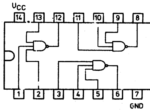
7410
