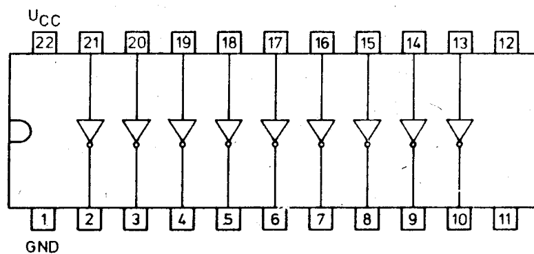
74548, 74549
