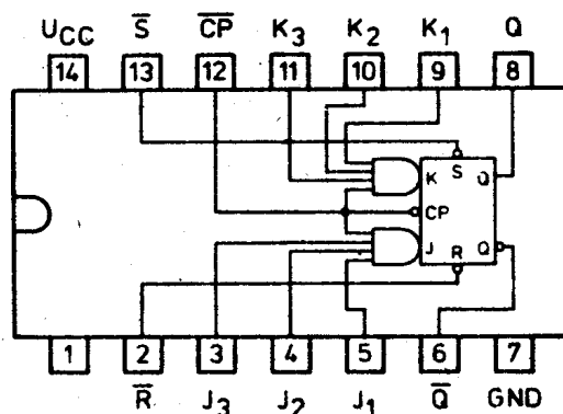
7472
