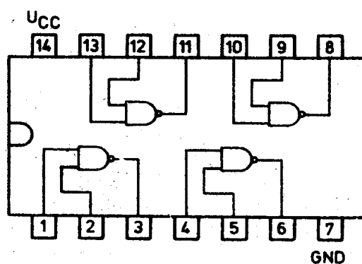
7437
