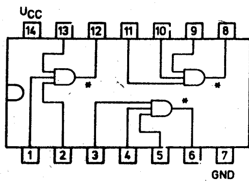
7415
