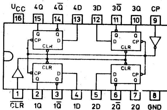
74175
