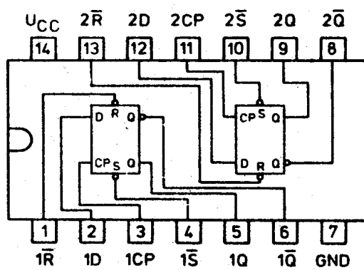
7474
