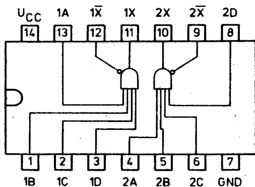
7460
