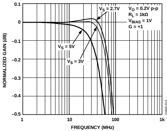
图14. 0.1 dB平坦度
