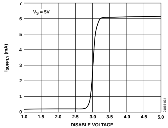
图34. AD8063 \overline{\text{DISABLE}} 电压与电源电流的关系
