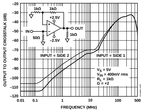
图32. AD8062串扰( V_{OUT} = 2.0\text{ V p-p} , R_L = 1\text{ k}\Omega , G = 2 , V_S = 5\text{ V} )
