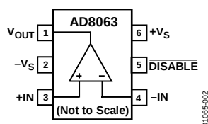
图3. 6引脚SOT-23 (RJ)
