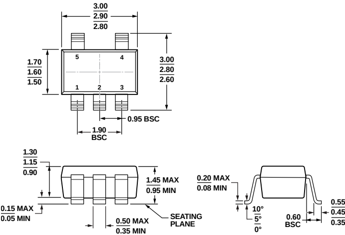
图58. 5引脚小型晶体管封装[SOT-23] (RJ-5)
