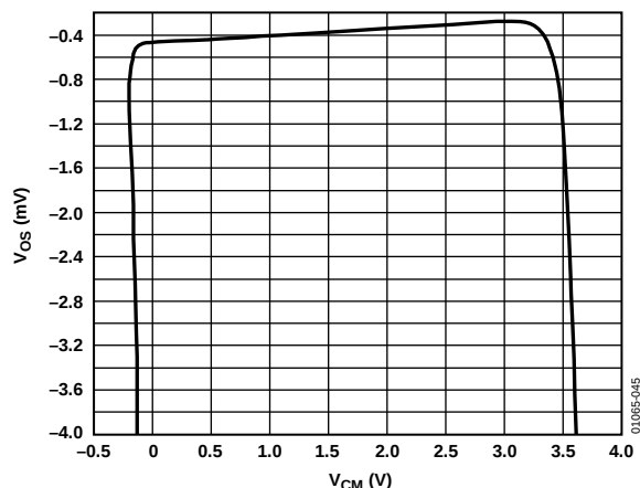
图45. V_{OS} 与共模电压的关系( V_S = 5 \text{ V} )
