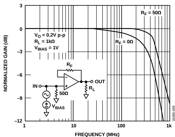
图5. 小信号响应, R_F = 0 \Omega , 50 \Omega
