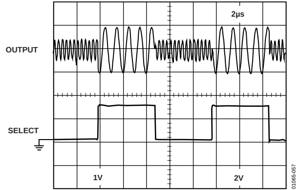
图57. AD8063多路复用器输出
