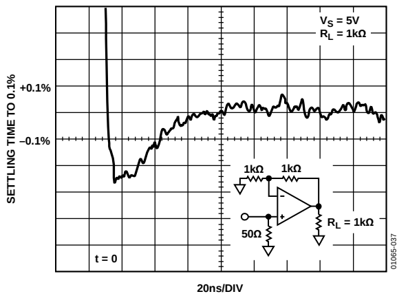
图37. 输出0.1%建立时间
