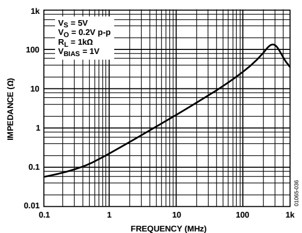
图36. 输出阻抗与频率的关系 ( V_{OUT} = 0.2\text{ V p-p} , R_L = 1\text{ k}\Omega , V_S = 5\text{ V} )
