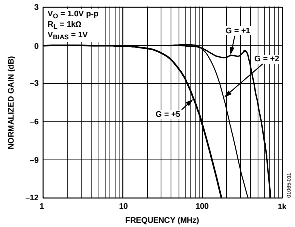
图11. 大信号频率响应
