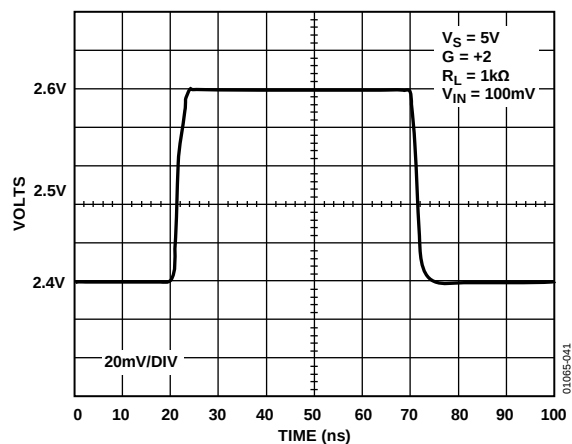
图41. 100 mV步进响应
