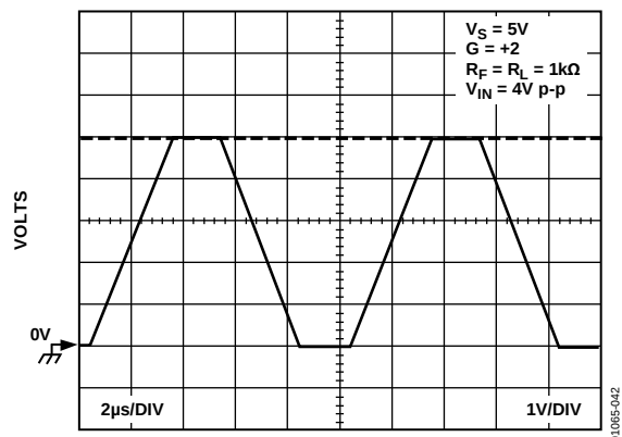
图42. 输出轨到轨摆幅
