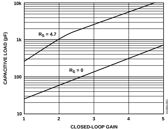
图51. 容性负载与闭环增益的关系
