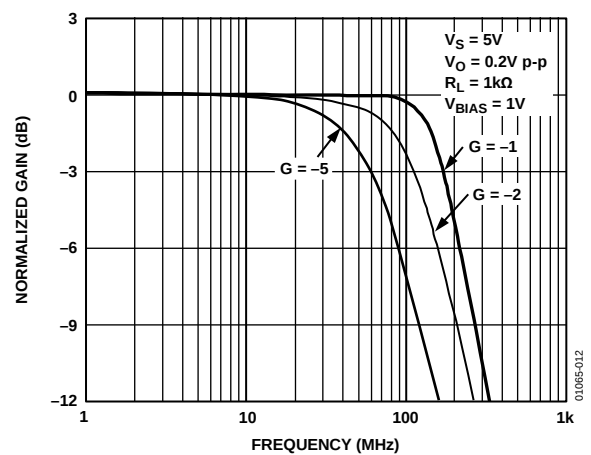
图12. 小信号频率响应
