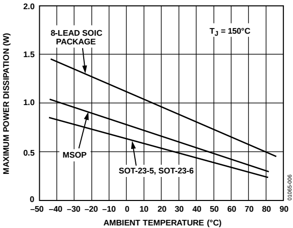
图6. AD8061/AD8062/AD8063 最大功耗与温度的关系
