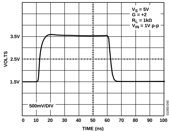
图40. 1 V步进响应
