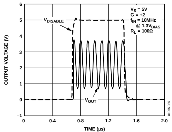
图35. AD8063 \overline{\text{DISABLE}} 功能(电压 = 0 V至5 V)
