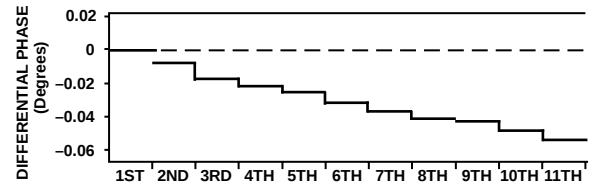
图22. 差分增益和相位误差 ( G = 2 , NTSC输入信号, R_L = 1k\Omega , V_S = 5V )
