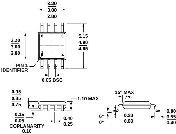
图61. 8引脚超小型封装[MSOP] (RM-8)
