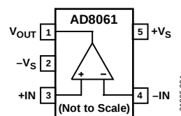
图4. 5引脚SOT-23 (RJ)
