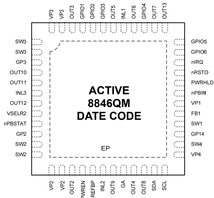
Thin - QFN (TQFN66-48)
