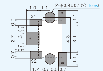
推奨はんだ付けパターン Recommendable soldering pattern (Top view)
