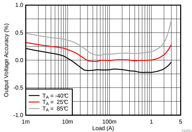
图 19. Load Regulation
