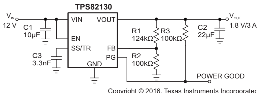
图 5. 1.8-V Output Application
