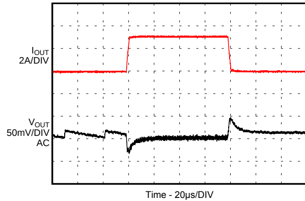
图 25. Load Transient
