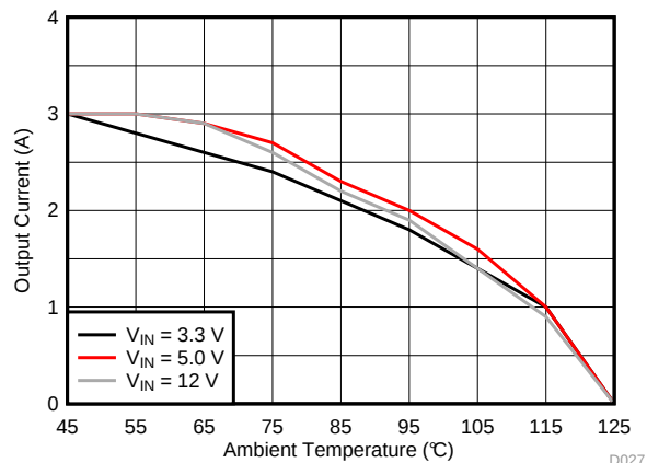
图 18. Thermal Derating, V_{OUT} = 1.0\text{ V}
