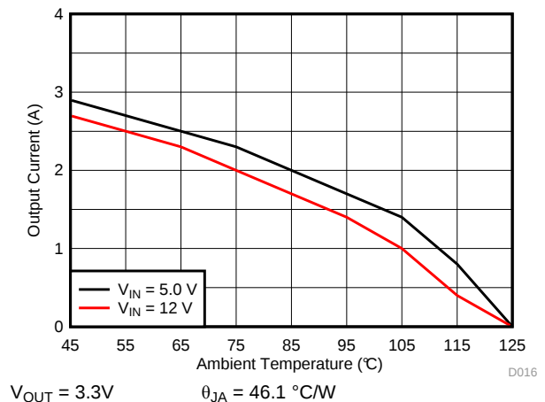
图 17. Thermal Derating, V_{OUT} = 3.3\text{ V}
