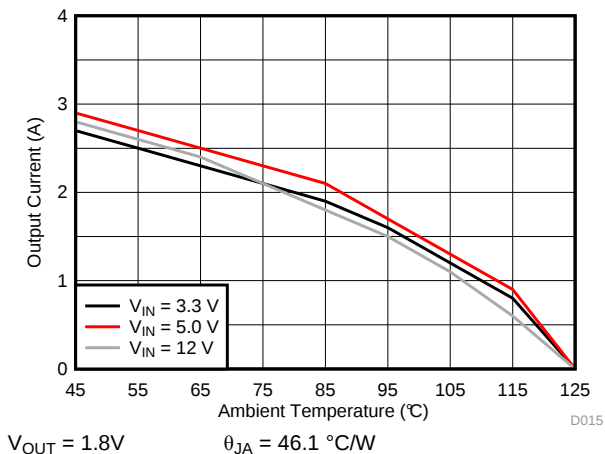
图 16. Thermal Derating, V_{OUT} = 1.8\text{ V}
