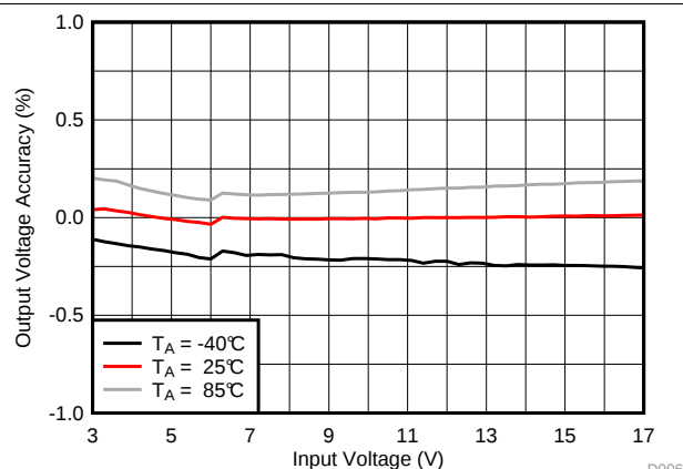
图 20. Line Regulation
