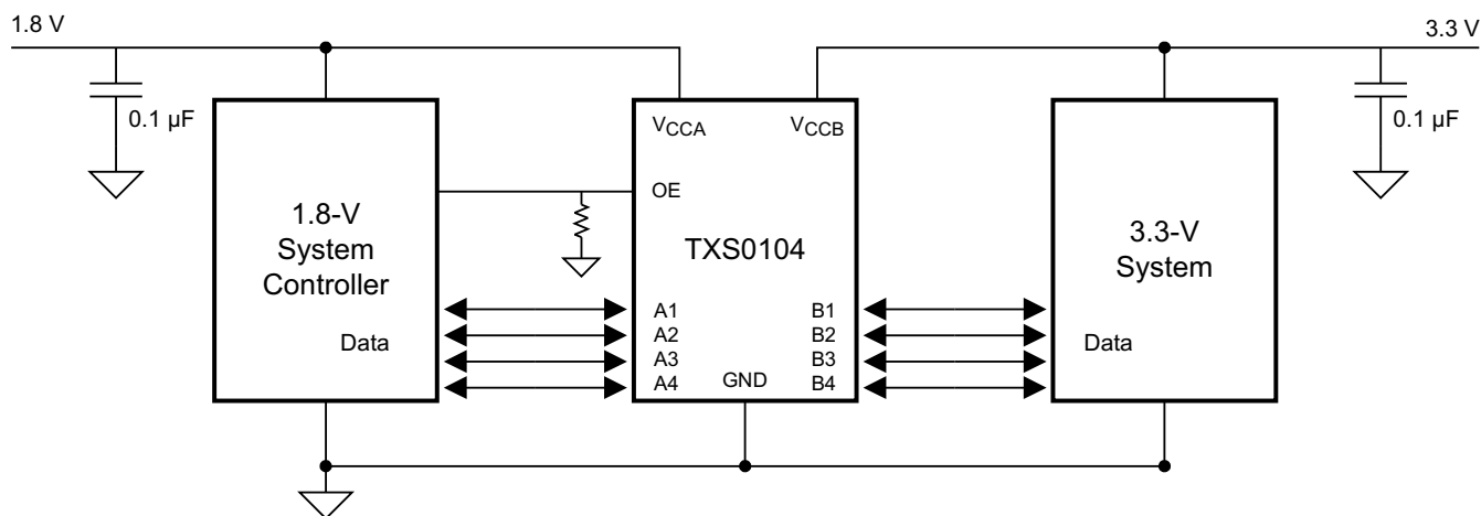
图 9-1. 应用原理图
