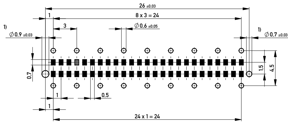
1) Durchmesser des Bohrers / drill tool
