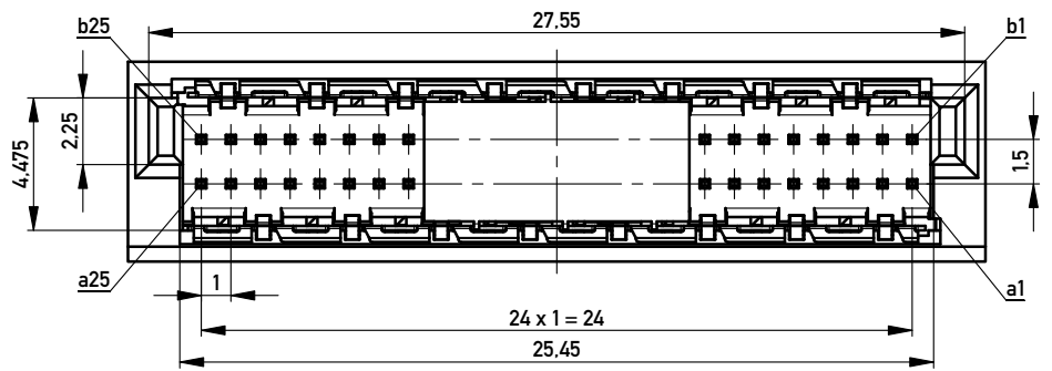
Leiterplatten-Layout Vorschlag / PCB-layout proposal
