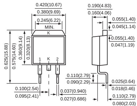
D2PAK
