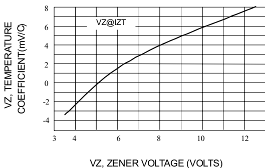
Fig. 7-ZENER VOLTAGE-TO 12 VOLTS
