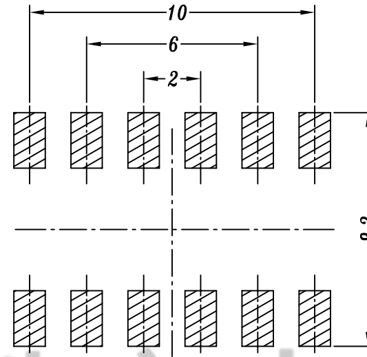
P.C.B LAYOUT
