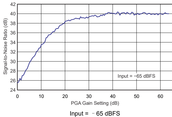
图 8-7. ADC SNR vs PGA Gain Setting, -65-dBFS Input
