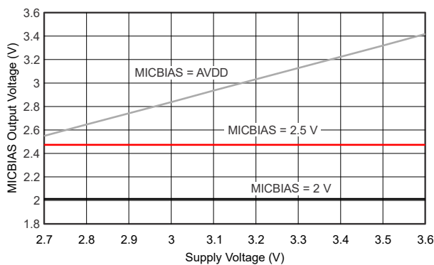
图 8-9. MICBIAS Output Voltage vs AVDD
