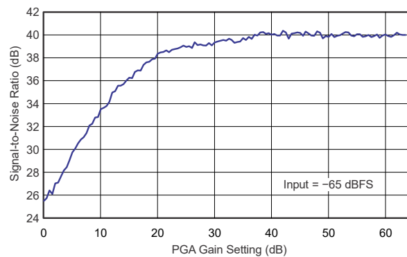
图 10-4. ADC SNR vs PGA Gain Setting, -65-dBfs Input
