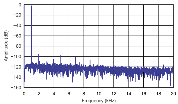
图 8-6. Line Input to ADC FFT Plot
