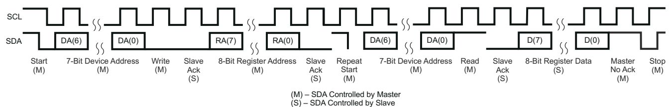
图 9-15. I 2 C Read
