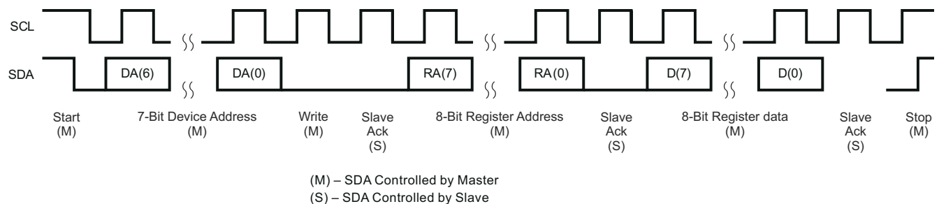
图 9-14. I 2 C Write
