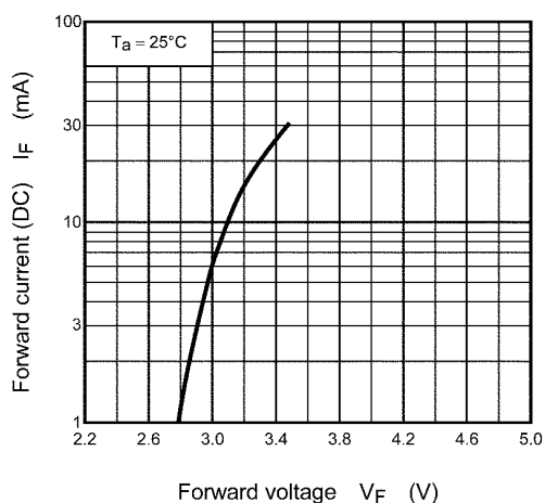
Fig. 8.1 I_F - V_F
