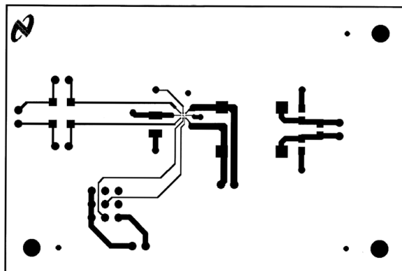
Top Layer
