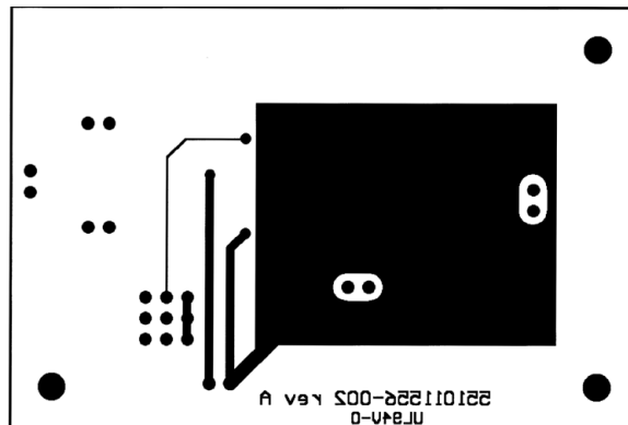
Bottom Layer
