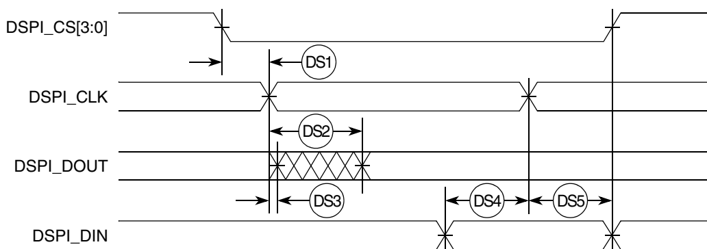
Figure 26. DSPI Timing
