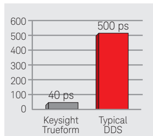
Jitter
