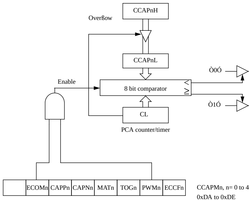
Figure 27. PCA PWM Mode
