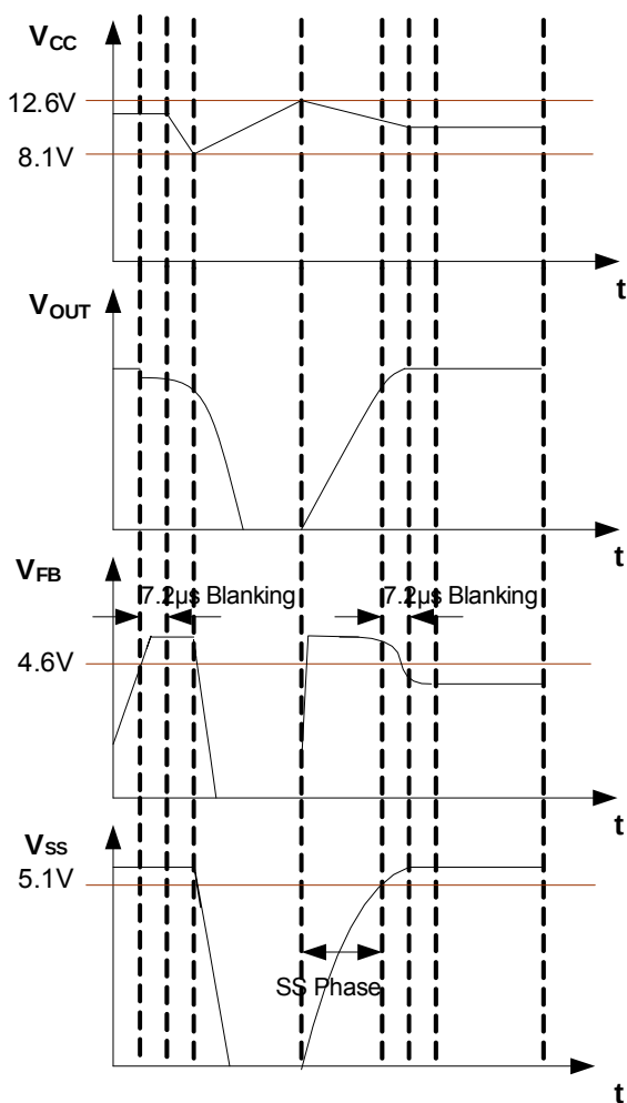
FIG.4 OLP case
