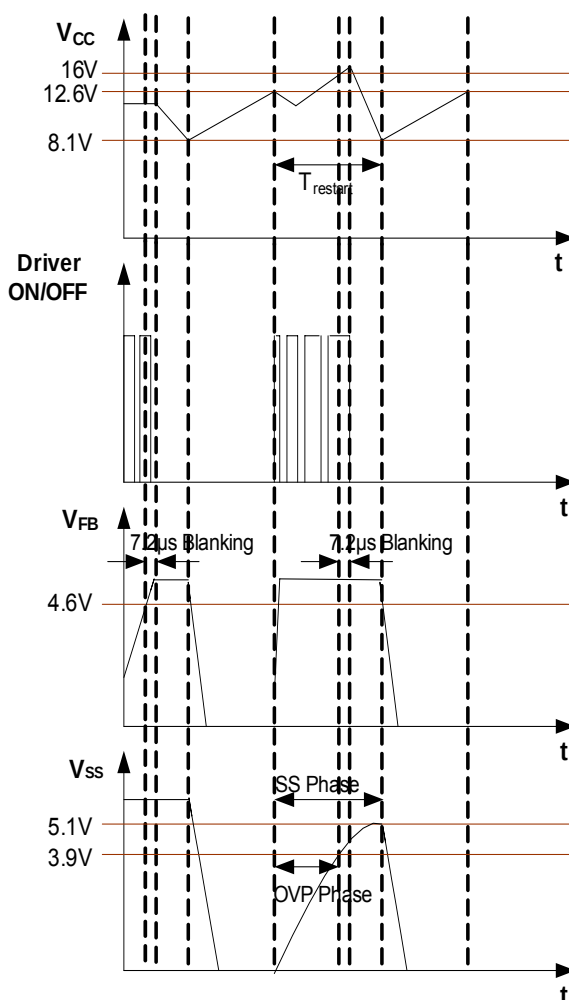
FIG.5 OVP case
