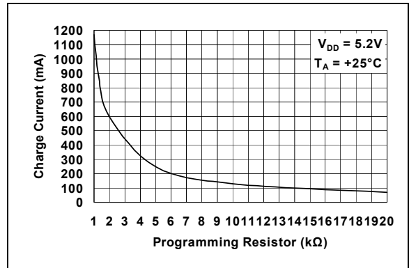
图 2-5: 充电电流 ( I_{OUT} ) — 可编程电阻 ( R_{PROG} )
