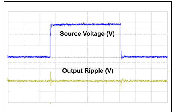
图 2-17： 线路瞬态响应 ( I_{LOAD} = 10 \text{ mA} ，输出：1.0V/Div，源电压：2.0V/Div)
