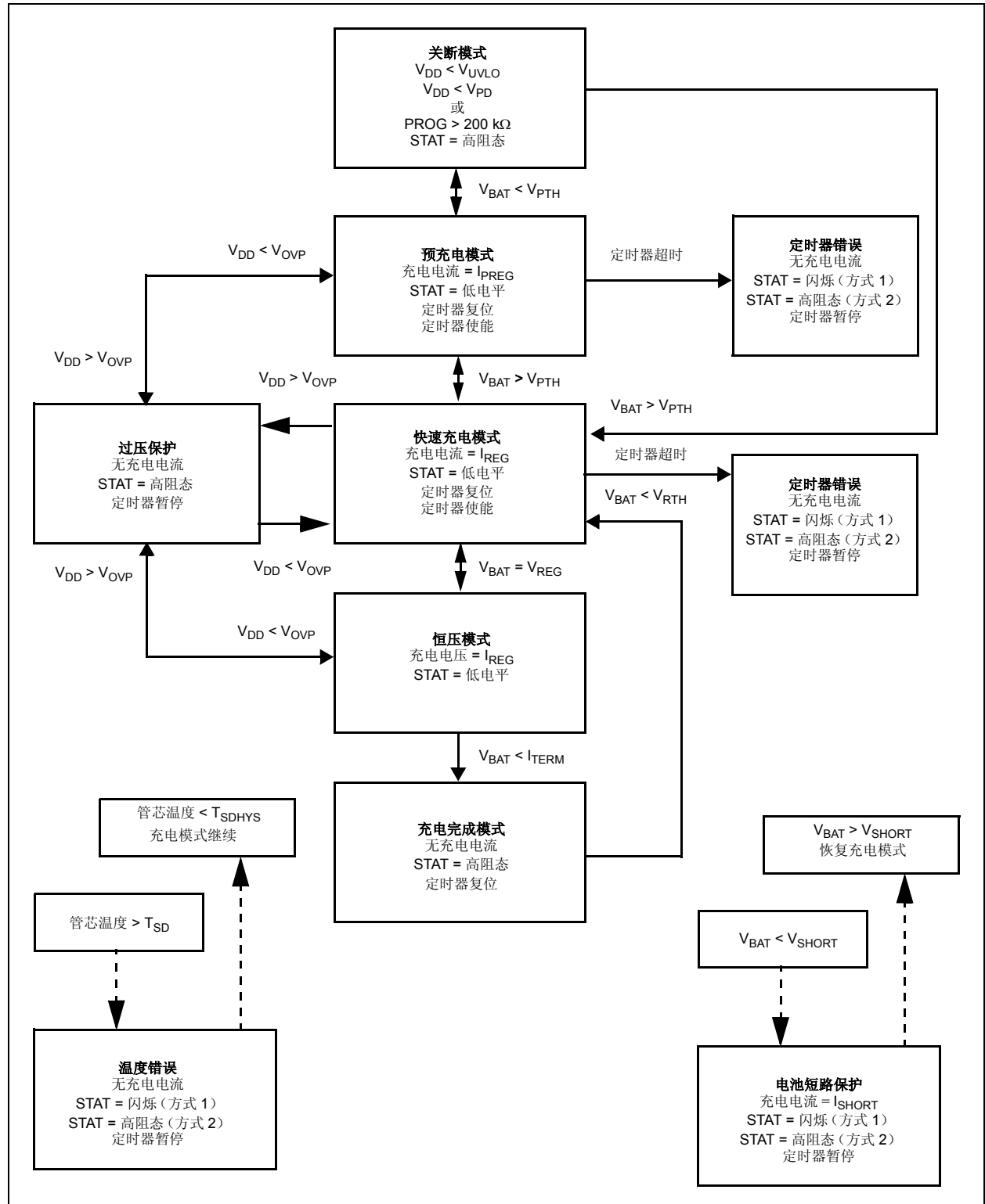
图 4-1: MCP73113/4 流程图
