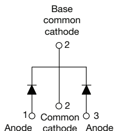
VS-10CTQ150-1-M3
