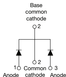
VS-10CTQ150S-M3
