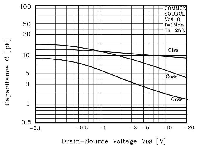
Fig6 C - V_{DS}
