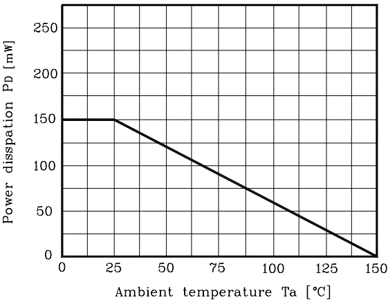
Fig9 Pd - Ta
