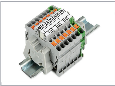
Beschriftungsstreifen (2009-110) eingesetzt in die Beschriftungsaufnahme mit Brückersymbolik des eingesetzten Brückers (Sternbrücker 2000-405/011-000) (hier am Beispiel Klemmen mit Drücker)
