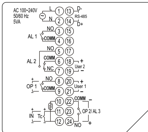
1/8 or 1/4 DIN
