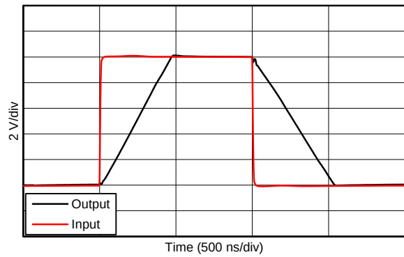
10V 阶跃 G = +1
