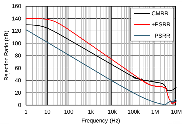
图 14. CMRR 和 PSRR 与频率间的关系
