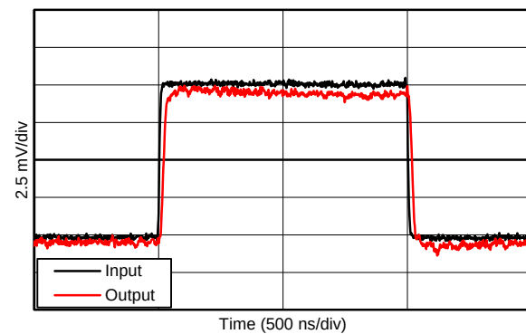
10mV 阶跃 G = +1
