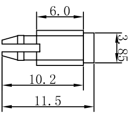
铆钉示意图
