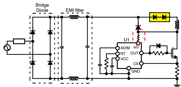
图 6. 高压应用
