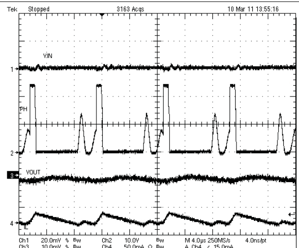
Figure 48. DCM 下的输入和输出纹波
