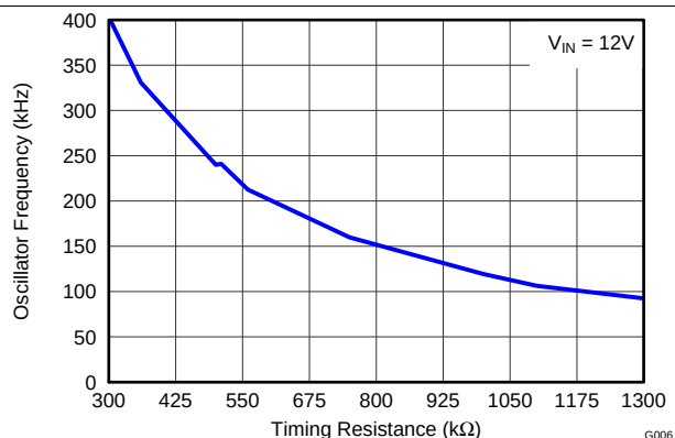
Figure 6. 频率与 R_T/CLK 电阻间的关系
