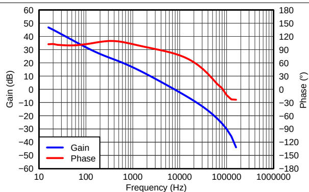
Figure 23. 增益与相位间的关系
