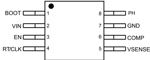
MSOP 封装 8 引脚 俯视图
