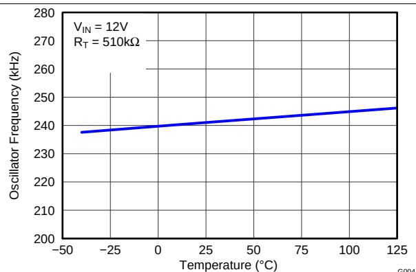
Figure 5. 频率与温度间的关系
