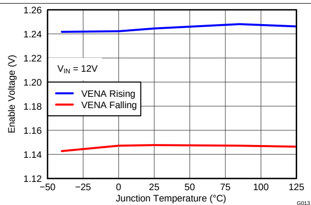
Figure 8. 使能引脚电压与温度间的关系
