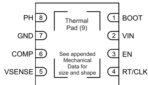
引脚功能
