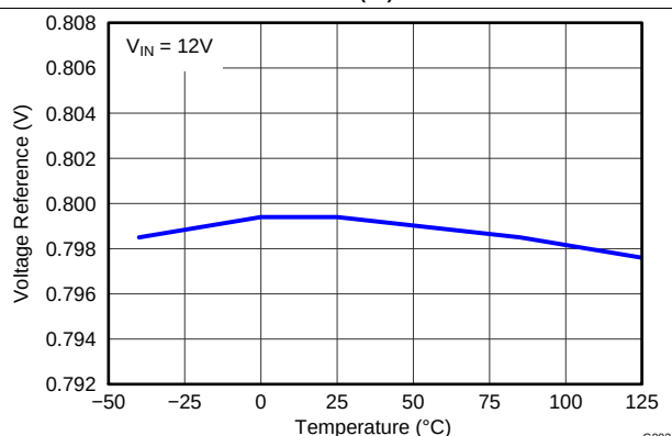
Figure 3. V_{REF} 电压与温度间的关系
