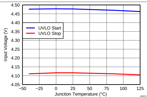
Figure 10. 输入电压 (UVLO) 与温度间的关系
