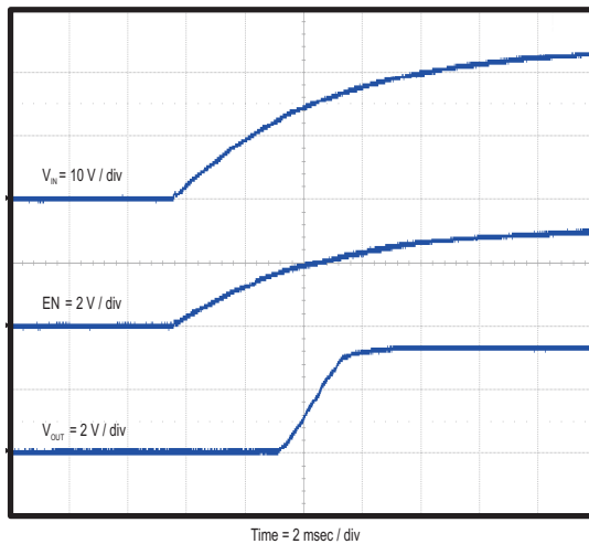
Figure 29. 以 V_IN 启动
