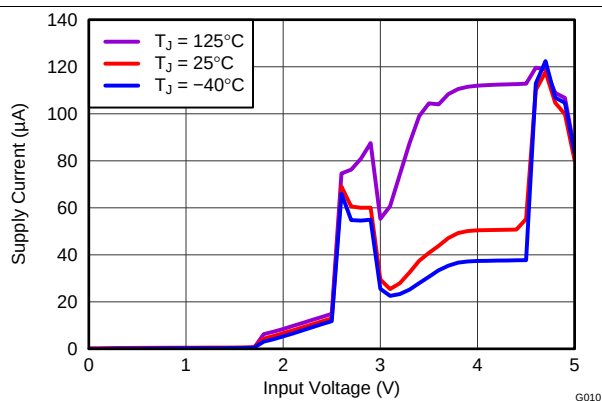
Figure 15. 电源电流 (VIN 引脚) 与输入电压 (0V 至 V_{\text{START}} ) 间的关系 (EN 引脚开路)
