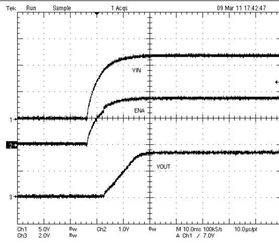
Figure 45. 以 V_{IN} 启动
