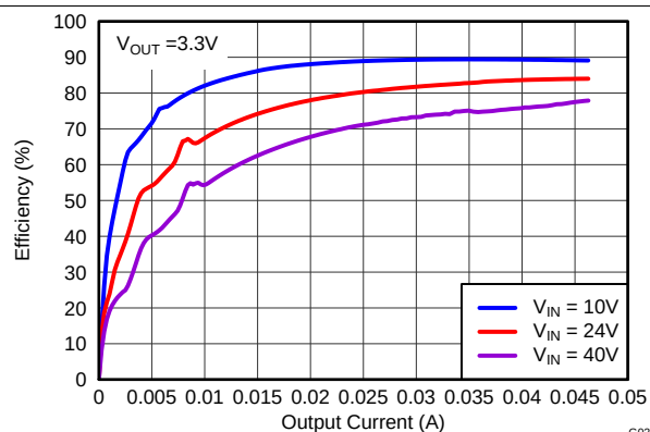
Figure 37. 效率与输出电流间的关系
