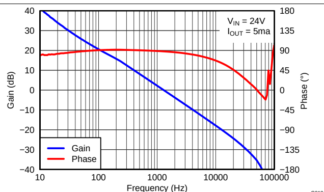
Figure 39. 增益与相位间的关系
