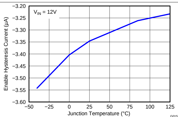
Figure 9. 使能引脚迟滞电流与温度间的关系
