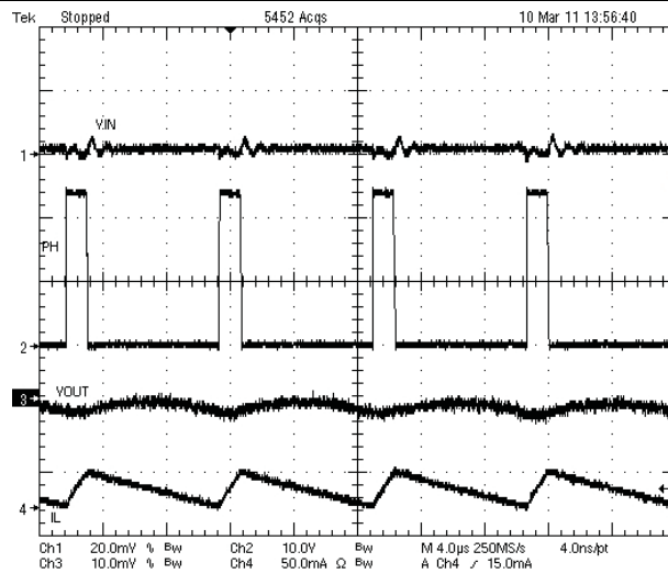
Figure 49. CCM 下的输入和输出纹波
