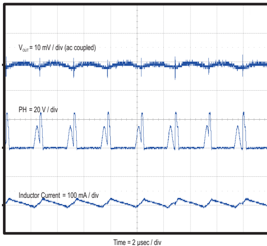
Figure 33. DCM 中的输出纹波
