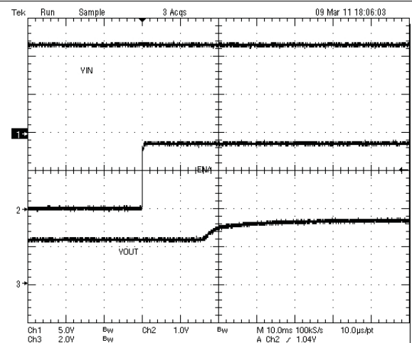
Figure 46. 以 ENA 预偏置启动
