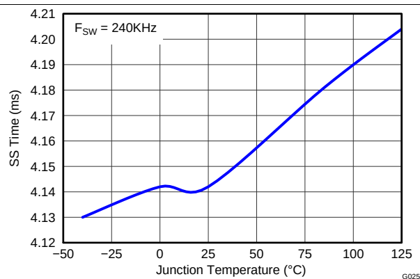
Figure 16. 缓慢启动时间与温度间的关系
