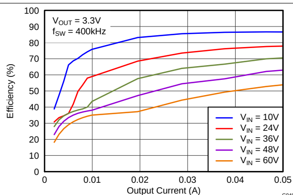
Figure 21. 效率与输出电流间的关系
