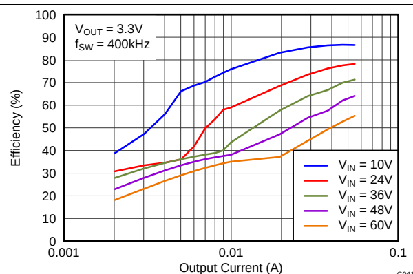
Figure 22. 效率与输出电流间的关系
