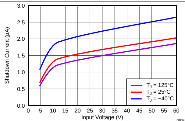
Figure 12. 关断电源电流 (VIN) 与输入电压间的关系
