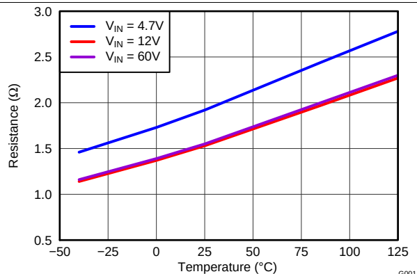
Figure 1. 高侧 R_{DS(on)} 与温度间的关系
