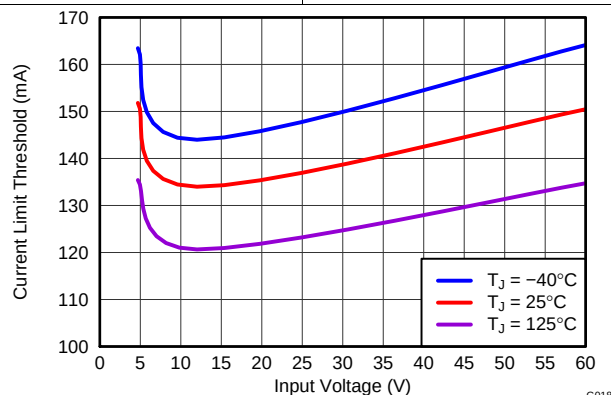
Figure 17. 电流限值 与输入电压间的关系
