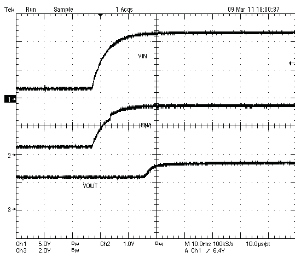
Figure 47. 以 V_{IN} 预偏置启动
