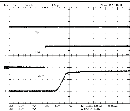
Figure 44. 以 ENA 启动
