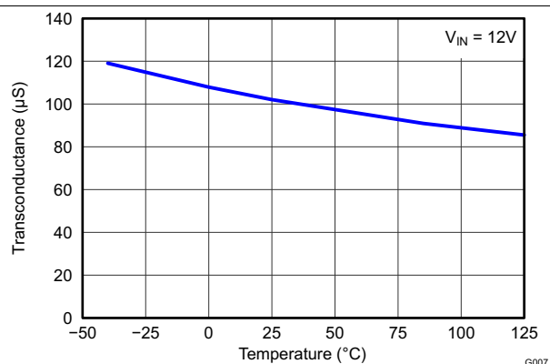
Figure 7. 误差放大器跨导与温度间的关系
