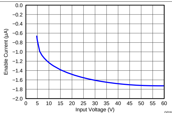
Figure 11. 使能引脚上拉电流与输入电压间的关系
