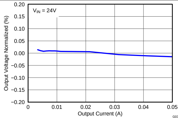
Figure 25. 输出电压与输出电流间的关系
