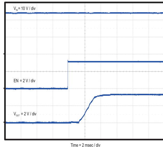
Figure 28. 以 ENA 启动
