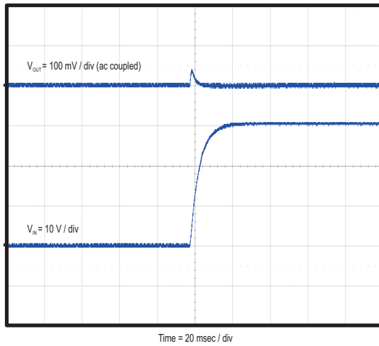
Figure 27. 线路瞬态
