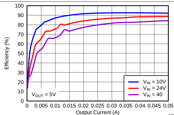
Figure 38. 效率与输出电流间的关系
