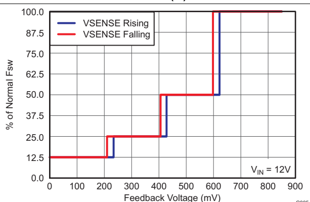
Figure 4. 频率与 V_{SENSE} 电压间的关系
