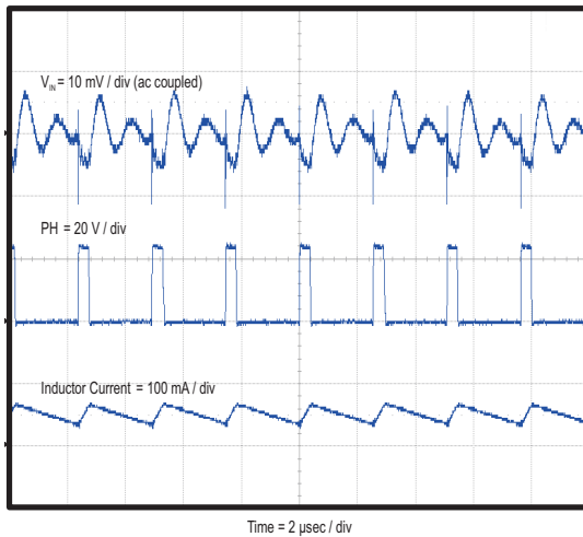
Figure 31. CCM 中的输入纹波
