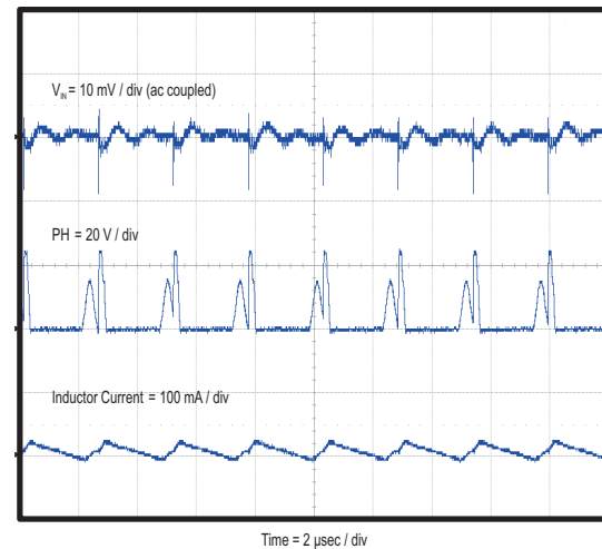
Figure 30. DCM 中的输入纹波
