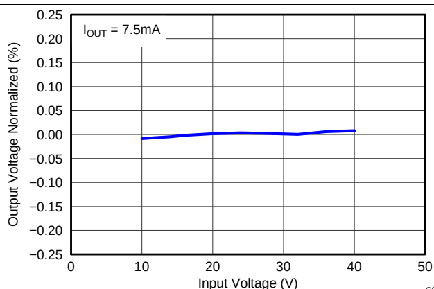
Figure 41. 静态电流与输入电压间的关系
