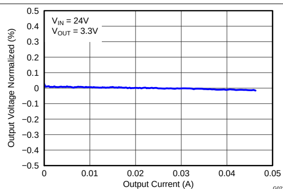
Figure 40. 输出电压与输出电流间的关系
