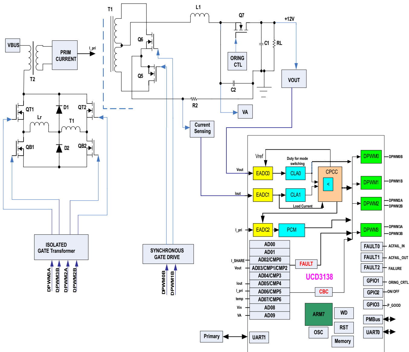
图 7-1. 相移全桥
