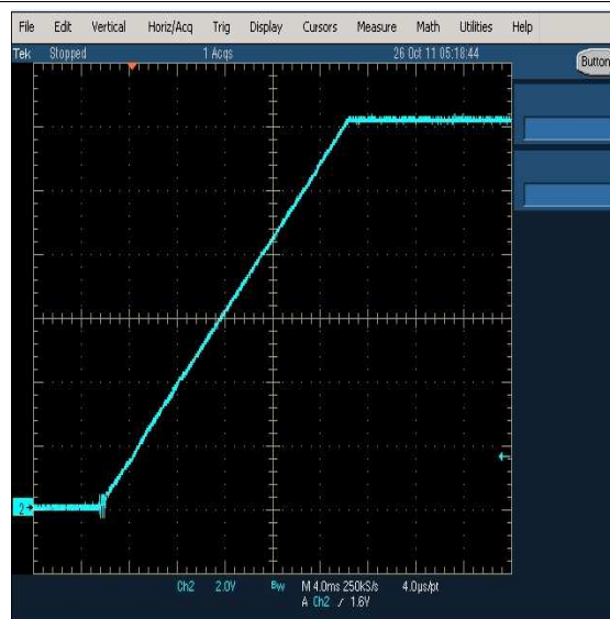
图 7-11. V_{OUT} 软启动
