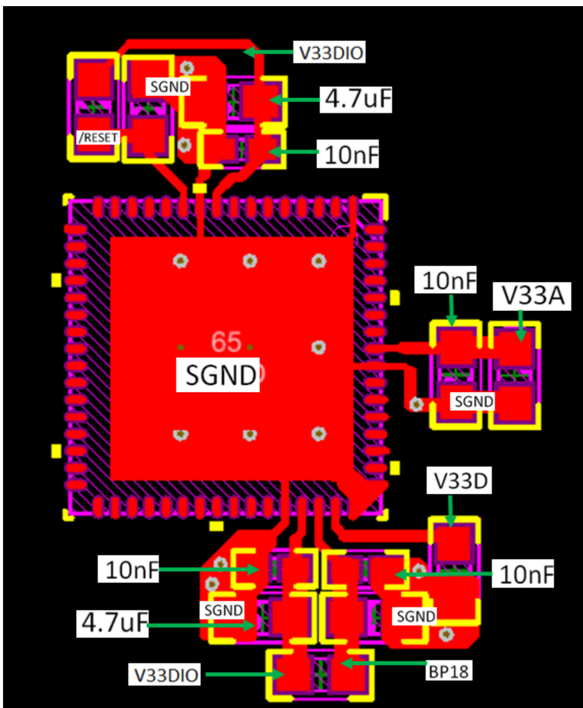
图 7-13. 布局示例
