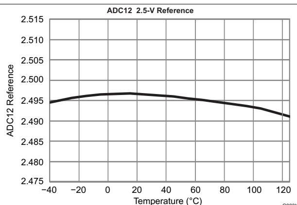
图 5-7. ADC12 2.5V 基准的温度变化图
