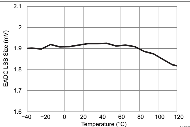
图 5-5. 具有 4 倍增益 (mV) 的 EADC LSB 大小的温度变化图
