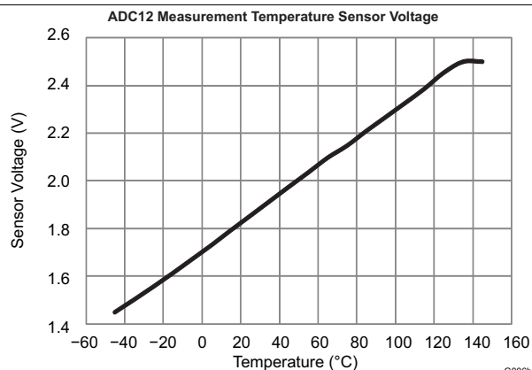
图 5-6. ADC12 测量温度传感器电压的温度变化图
