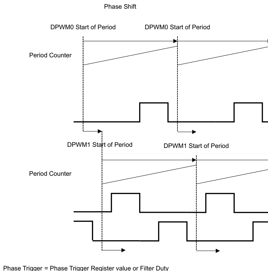
图 6-23. 相移
