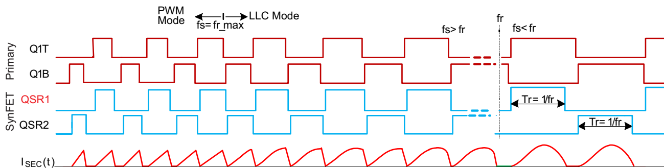
图 6-6. LLC 波形
