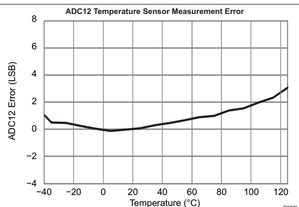
图 5-8. ADC12 温度传感器测量误差的温度变化图
