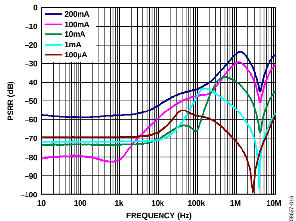
图18. 电源抑制比与频率的关系( V_{\text{OUT}} = 2.8\text{ V} , V_{\text{IN}} = 3.3\text{ V} )
