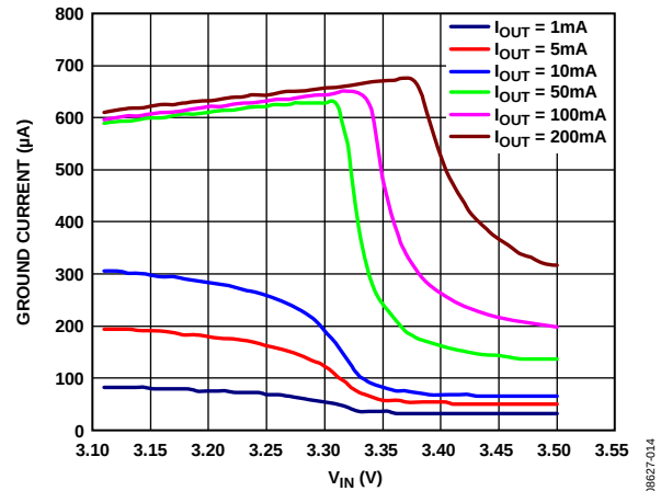
图16. 低压差下接地电流与输入电压的关系
