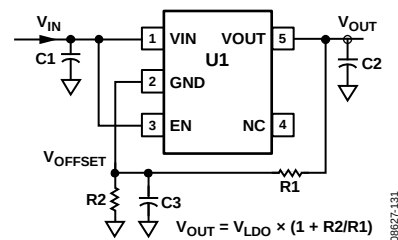
图33. 采用ADP151的可调LDO
