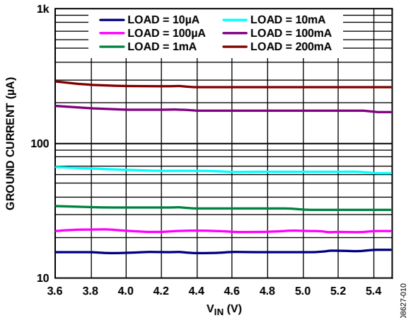
图12. 接地电流与输入电压的关系
