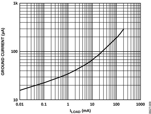
图11. 接地电流与负载电流的关系
