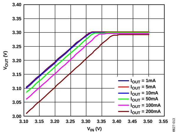
图15. 低压差下输出电压与输入电压的关系
