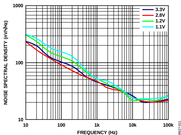
图23. 输出噪声谱密度与频率的关系 ( V_{IN} = 5\text{ V} , I_{LOAD} = 10\text{ mA} , C_{OUT} = 1\text{ μF} )
