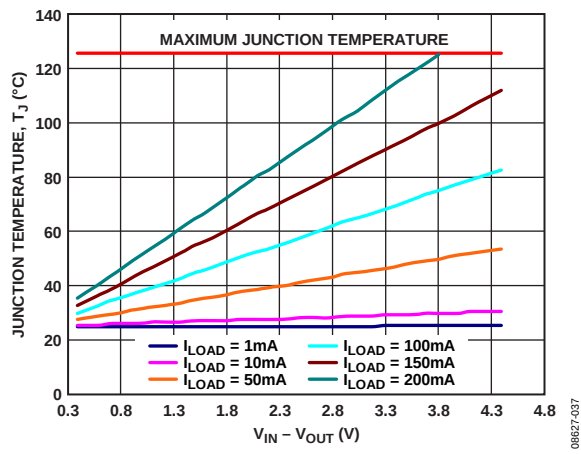
图45. TSOT 500 mm² PCB覆铜, T_A = 25^\circ C
