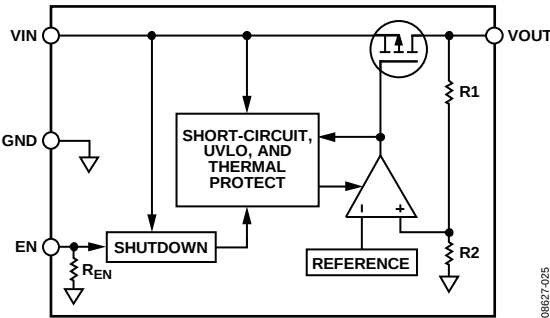
图27. 内部框图
