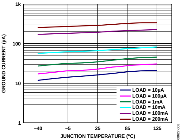
图10. 接地电流与结温的关系
