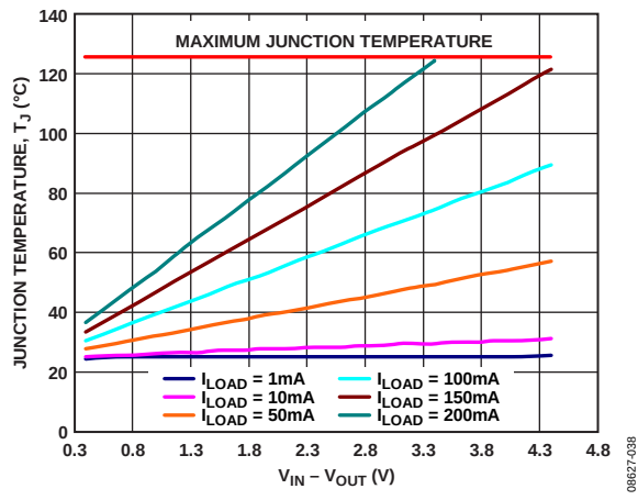
图46. TSOT 100 mm² PCB覆铜, T_A = 25^\circ C
