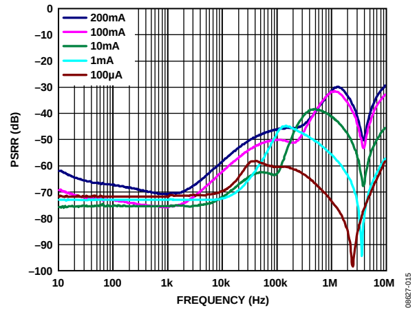
图17. 电源抑制比与频率的关系( V_{\text{OUT}} = 1.2\text{ V} , V_{\text{IN}} = 2.2\text{ V} )
