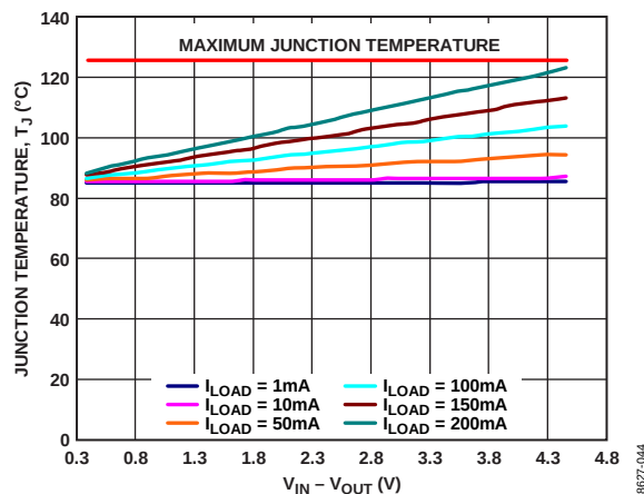
图58. TSOT封装, T_A = 85^\circ\text{C}
