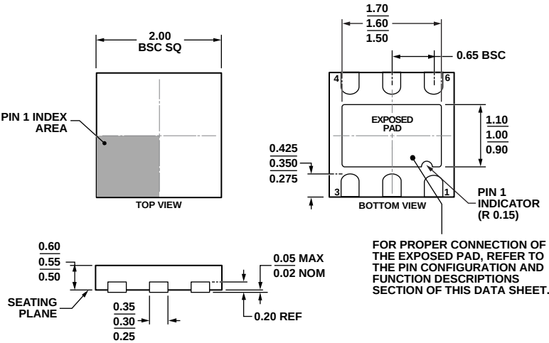
图65. 6引脚引脚架构芯片级封装 [LFCSP_UD] 2.00 mm x 2.00 mm超薄体双引脚(CP-6-3) (尺寸单位: mm)
