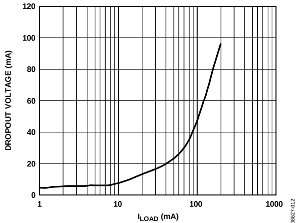
图14. 压差与负载电流的关系
