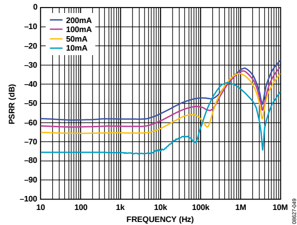
图37. 4 V LDO电路(典型PSRR与负载电流的关系, 电压裕量为1 V)
