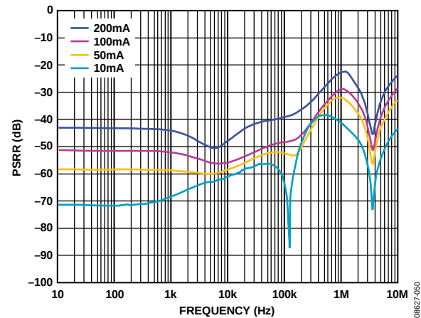
图38. 4 V LDO电路(典型PSRR与负载电流的关系, 电压裕量为500 mV)
