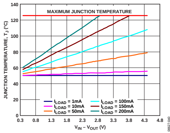
图48. TSOT 500 mm² PCB覆铜, T_A = 50^\circ C
