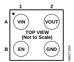
图5. 4引脚WLCSP引脚配置
