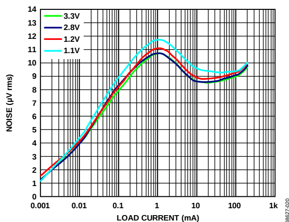
图22. 输出噪声与负载电流和输出电压的关系 ( V_{IN} = 5\text{ V} , C_{OUT} = 1\text{ μF} )
