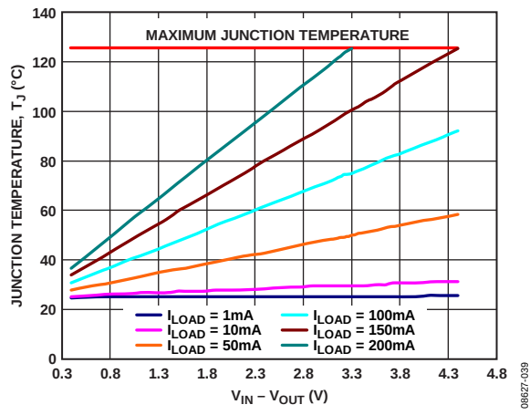
图47. TSOT 50 mm² PCB覆铜, T_A = 25^\circ C
